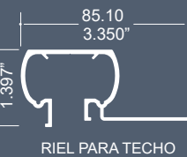
RIEL PARA TECHO
