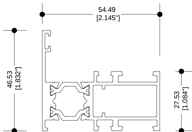
R007 CONTRAMARCO RPT
