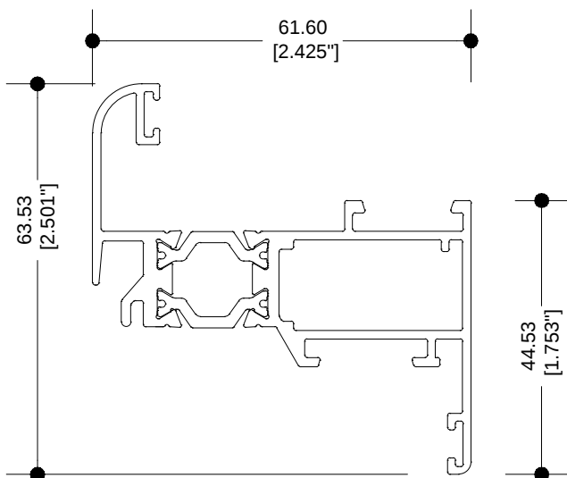
R008 "Z" APERTURA INTERIOR RPT
