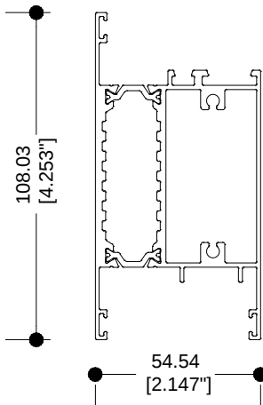
R016 ZOCLO
