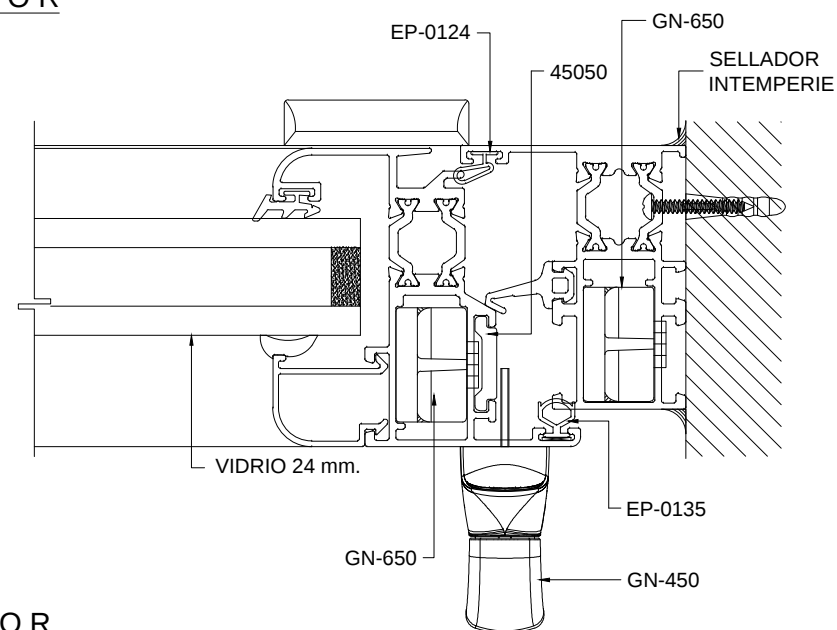
SECCIÓN 2
