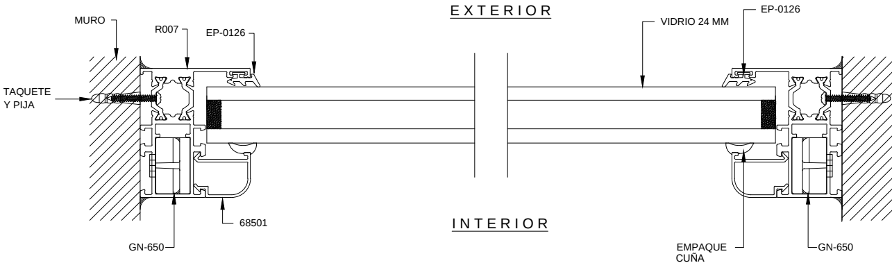
SECCIÓN 3
