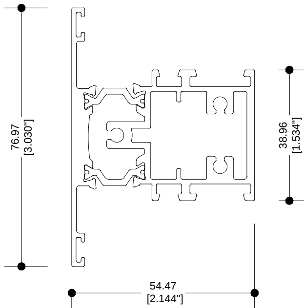
R020 RPT INTERMEDIO
