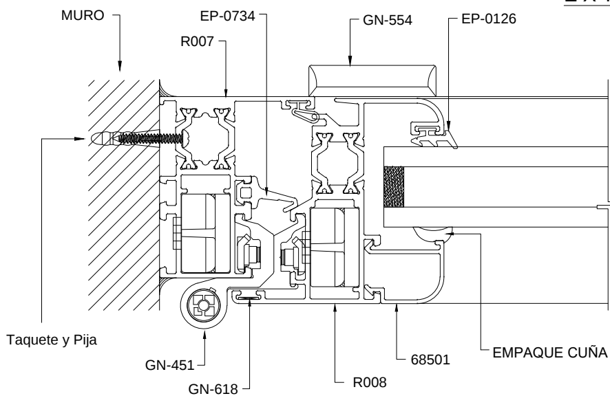
SECCIÓN 1
