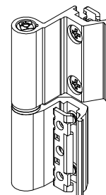
BISAGRA FLASH GN-451 PREMONTADA DERECHA CARACTERÍSTICAS: CAPACIDAD DE CARGA CON 2 BISAGRAS 75 KG. CON 3 BISAGRAS 85 KG. (CONSIDERANDO DIMENSIONES DE 1000 MM. x 2000 MM.)
