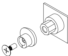
BULÓN DE CIERRE REGULABLE BT GN-479
