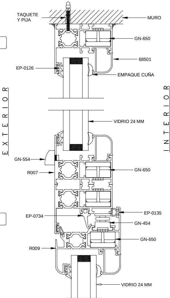
SECCIÓN 1
