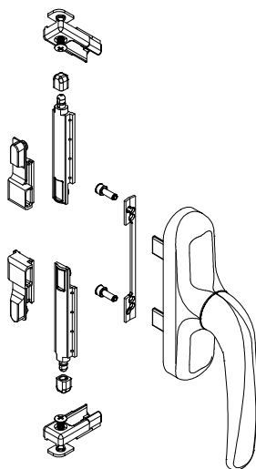
KIT CREMONA PRIMA GN-450 FUNCIÓN REVERSIBLE
