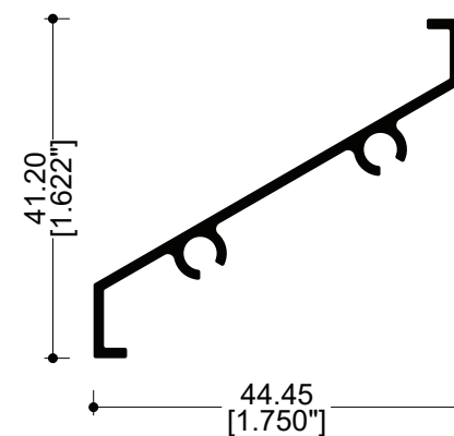
010088 Celosía fija
