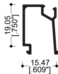
012543 Junquillo
