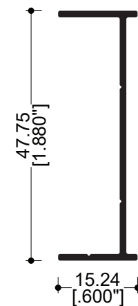
074268 Perfil celosía
