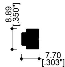
14412 Conector
