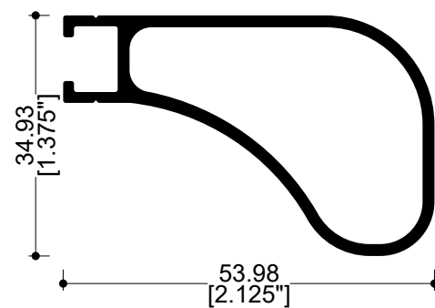
62014 Refuerzo
