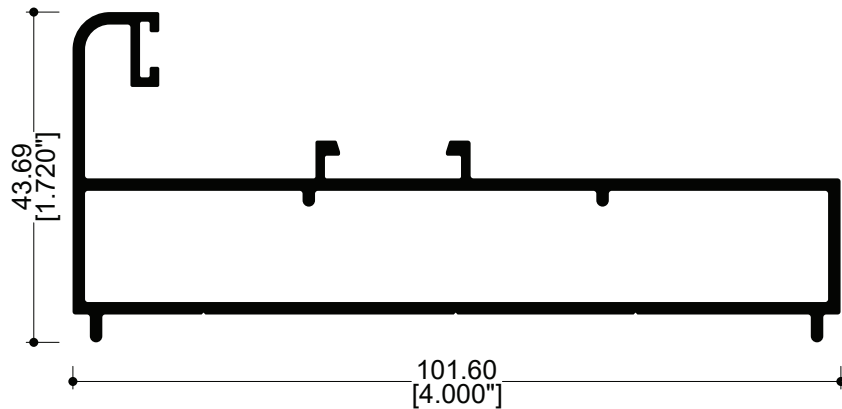
87734 Fijo 4"
