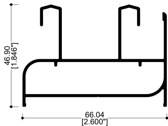
82000 Marco 2 vías
