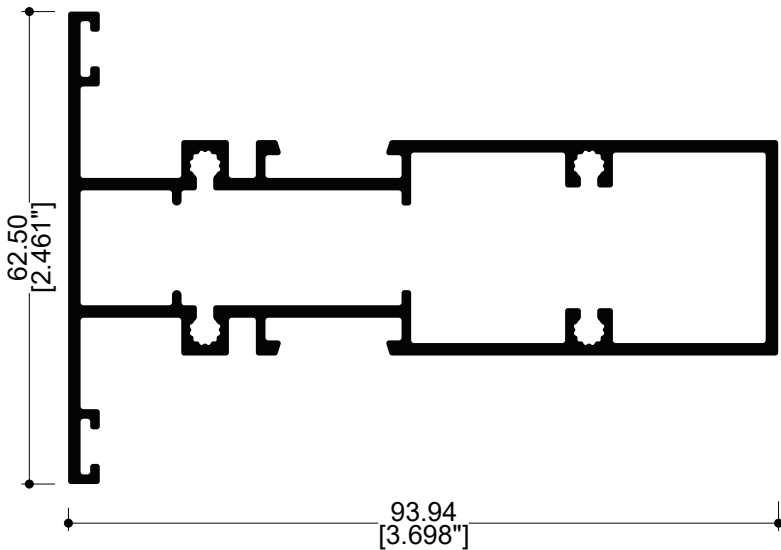
82047 Intermedio reforzado
