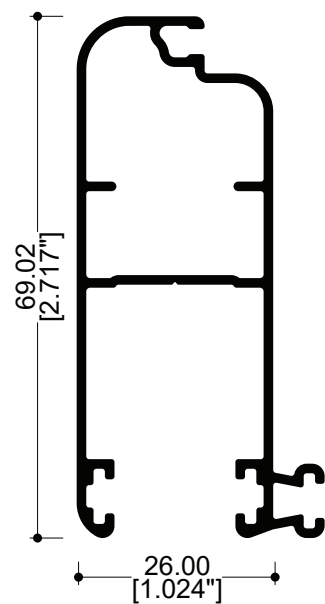
82019 Mosquitero
