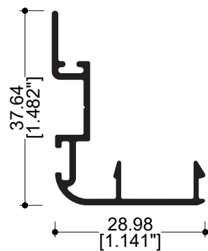
82002 Traslape
