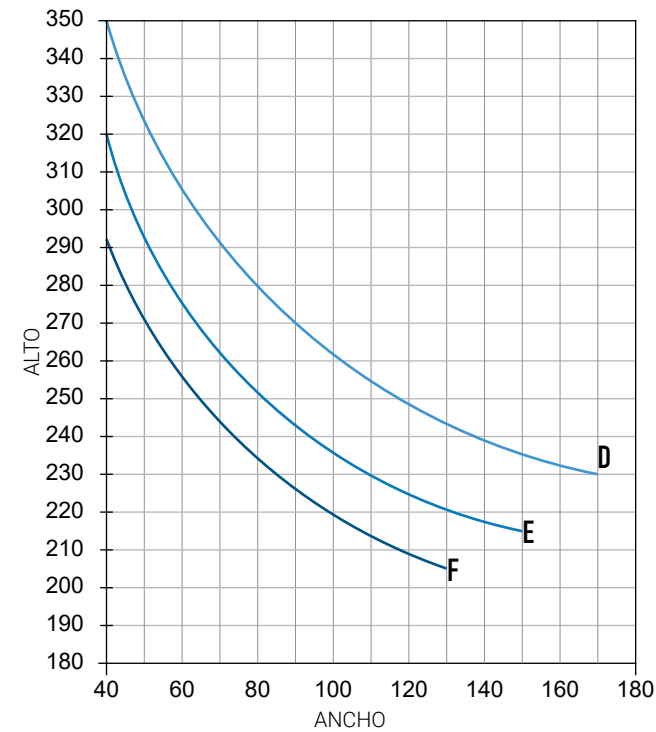
A UNA ALTURA DE 15 METROS DEFLEXIÓN MÁX. L/175
