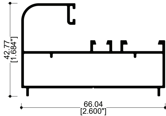
82092 Fijo
