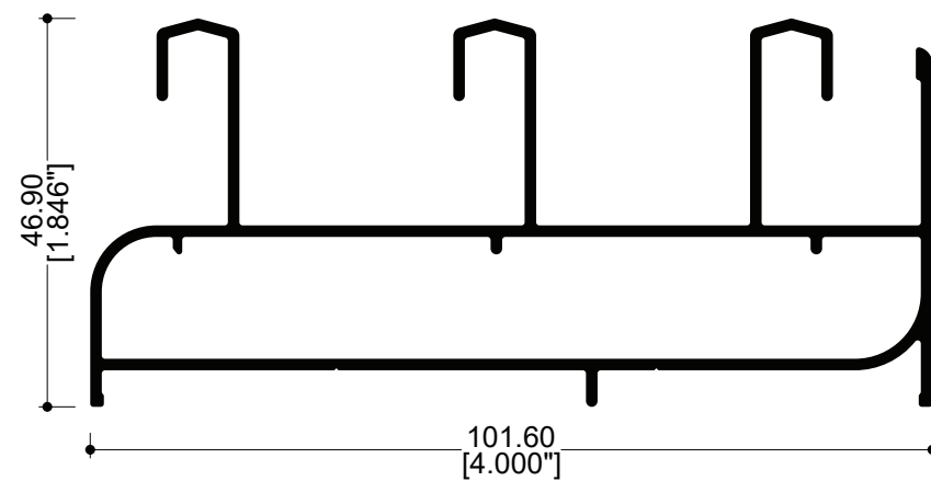
82017 Marco 3 vías
