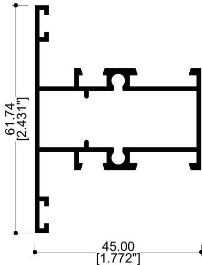
62041 Intermedio
