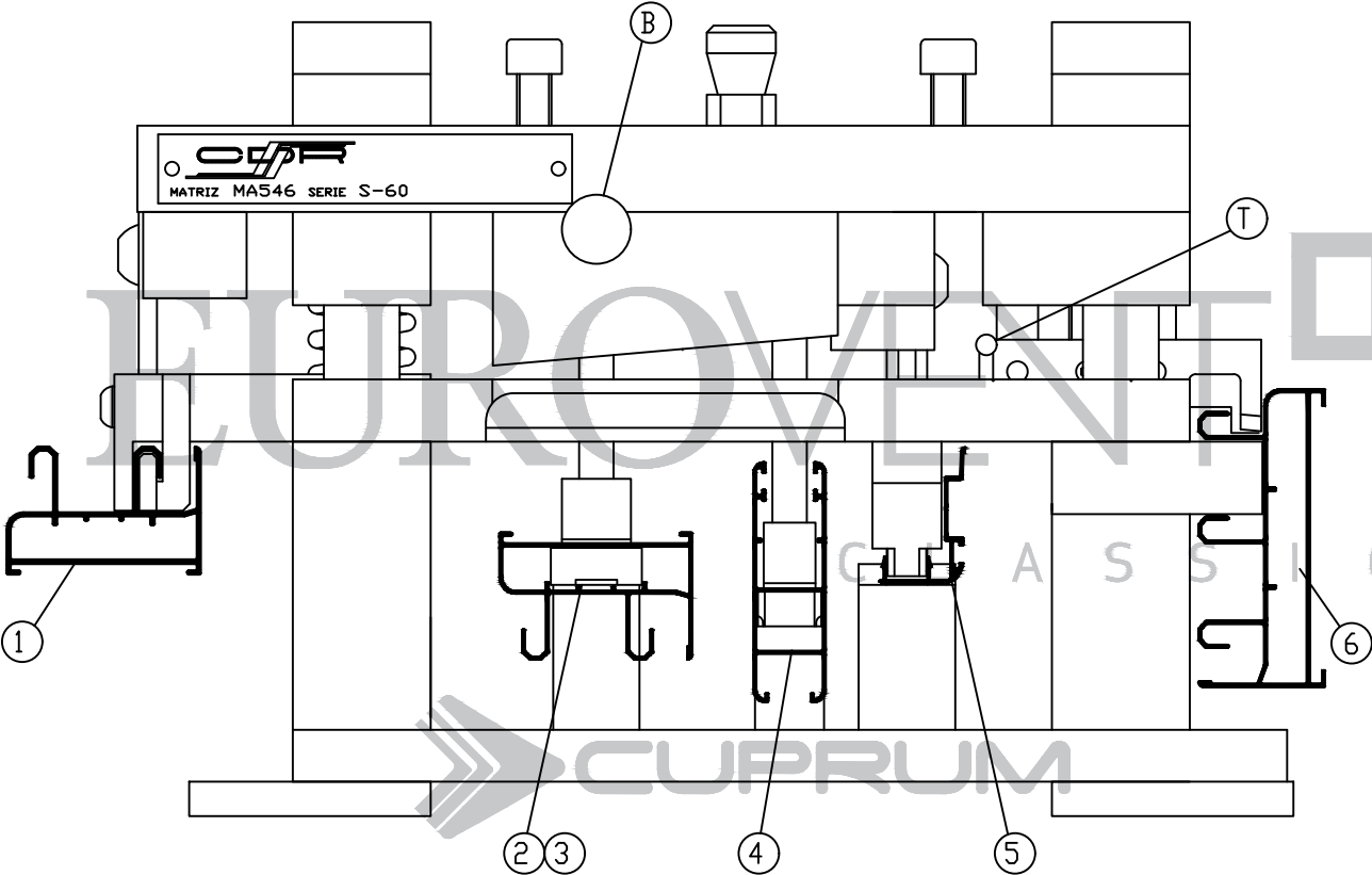
TROQUEL GN-533CDR VISTA FRONTAL
