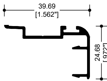
67899 TRASLAPE PUERTA
