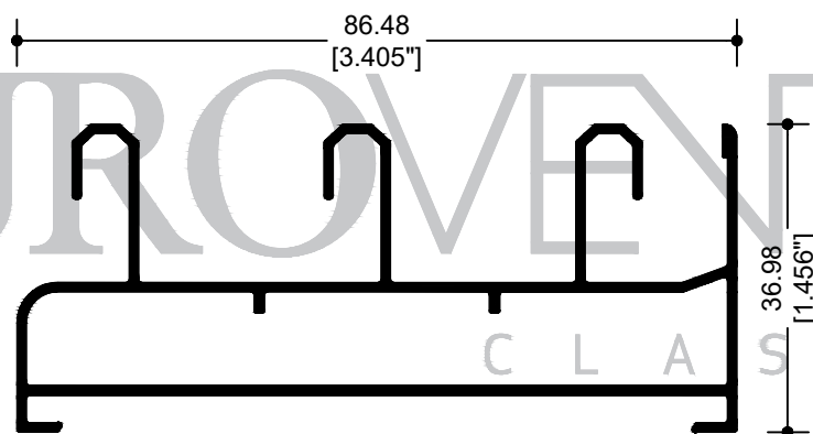
68300 RIEL TRIPLE
