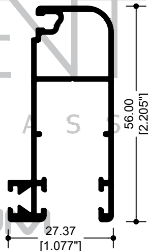
68337 MOSQUITERO VENTANA
