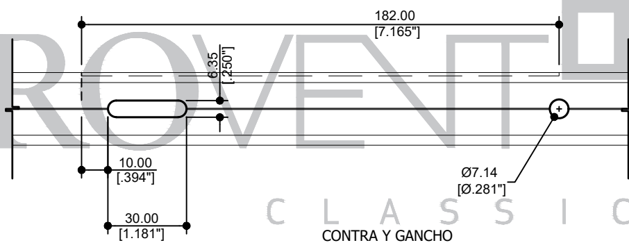
MEDIDA DEL CIERRE
