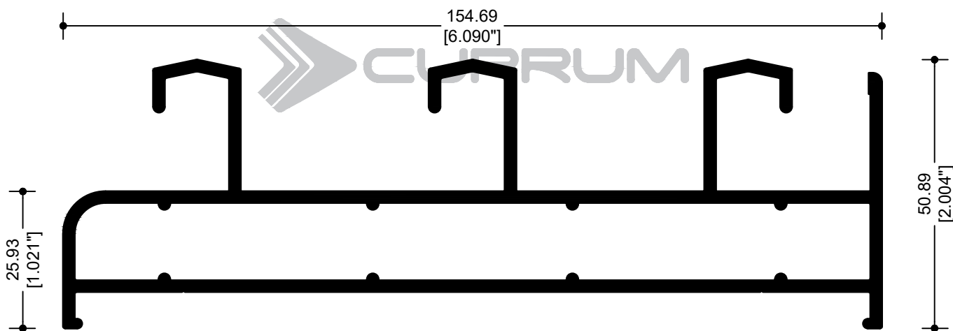
62054 RIEL TRIPLE
