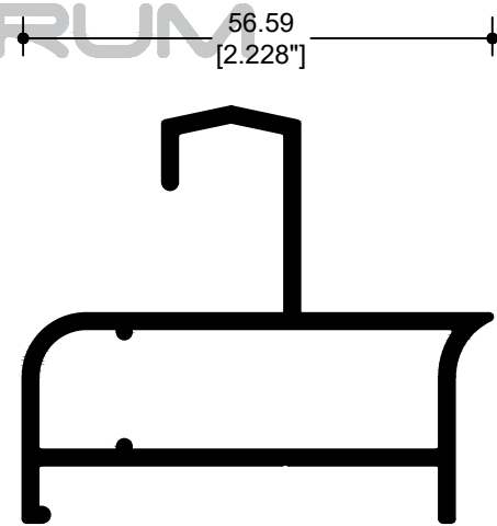
62091 ADAPTADOR RIEL
