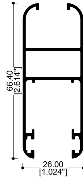
62001 Cercos 6 mm
