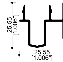
62103 Adaptador OXXO
