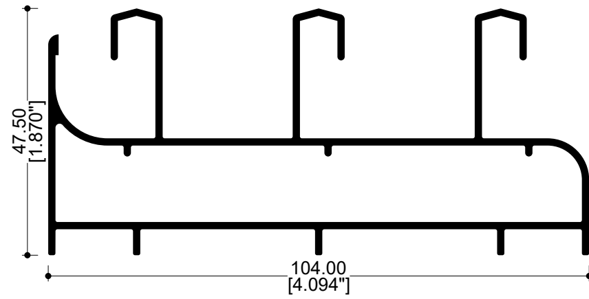
62017 Riel triple
