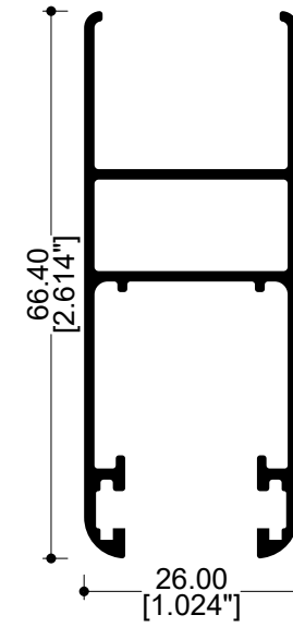
62004 Cercos 18 mm
