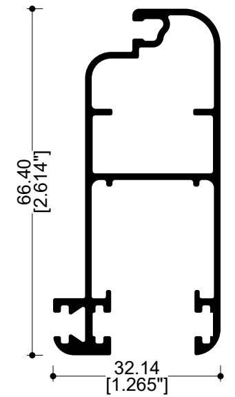
62019 Mosquitero
