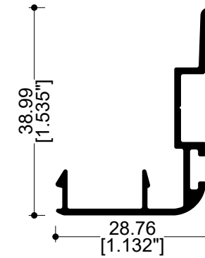
62002 Traslape
