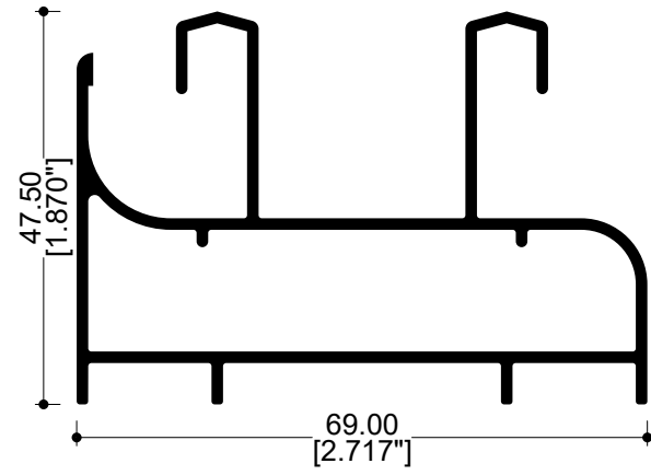
62000 Riel básico
