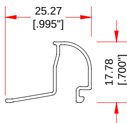
AB JUNQUILLO CONCAVO DOBLE
