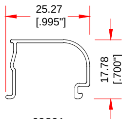
AB JUNQUILLO CONCAVO SENCILLO
