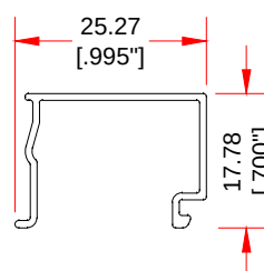
AB JUNQUILLO CUADRADO SENCILLO
