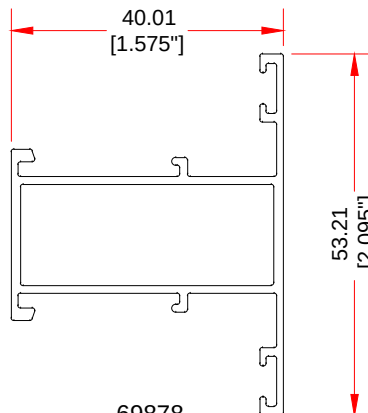
AB HOJA EXTERIOR VENTANA
