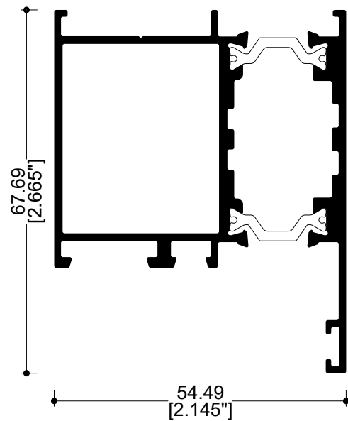
R028 Marco de puerta batiente
