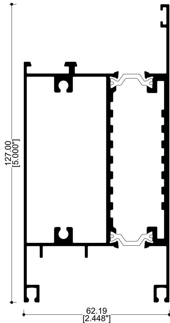
R029 Zoclo puerta batiente
