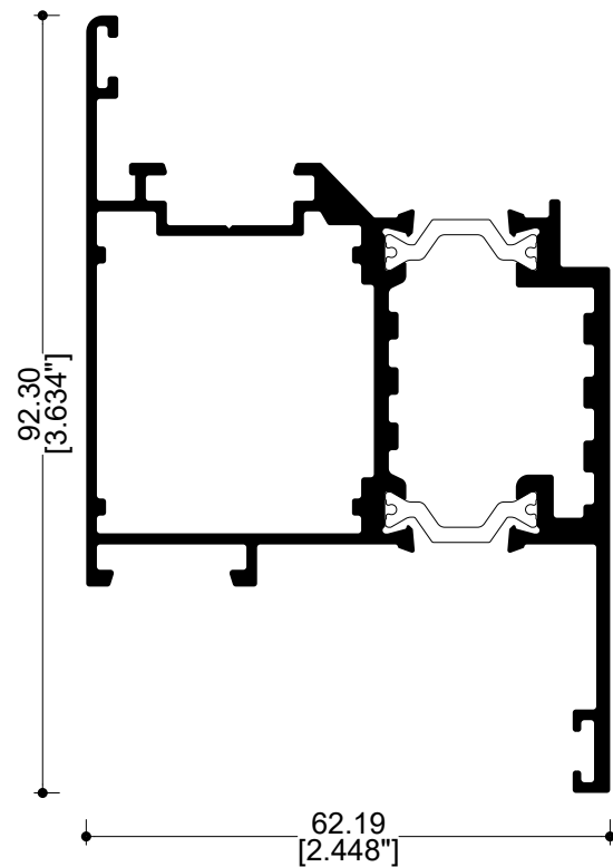
R027 Hoja puerta batiente
