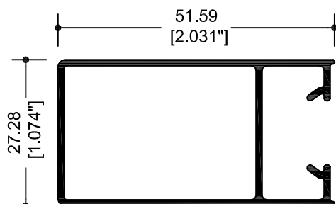
67847 CERCO CHAPA PUERTA
