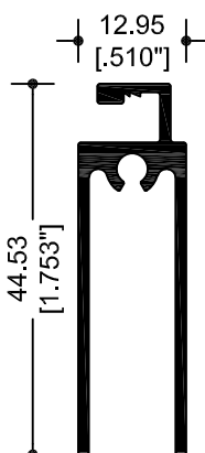
7104 MOSQUITERO
