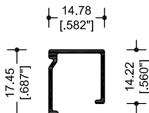
36370 JUNQUILLO
