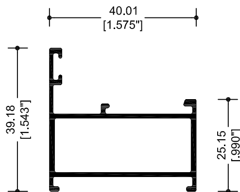
69877 MARCO VENTANA
