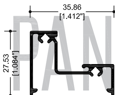
39074 ESCALONADO
