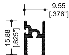
10575 ZOCLO
