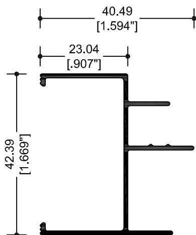
10570 JAMBA
