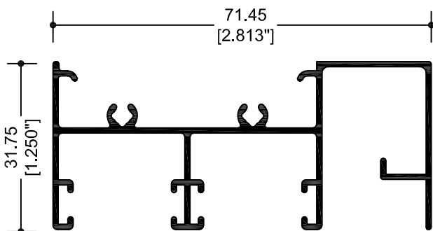
67819 CABEZAL MOSQUITERO COLGANTE
