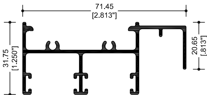
27819 CABEZAL MOS. CORREDIZO
