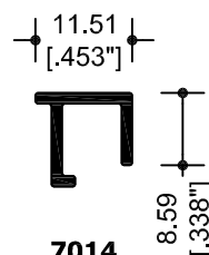
7014 JUNQUILLO
