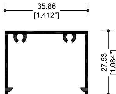
29076 BOLSA LISA
