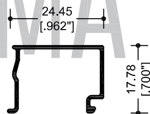
69890 JUNQUILLO CUADRADO SENCILLO (6mm)
