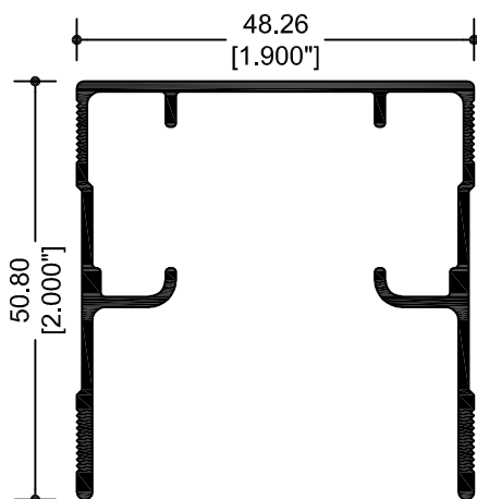
9947 RIEL SUPERIOR
