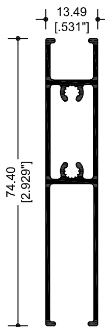
37825 ZOCLO PUERTA
