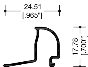
69887 JUNQUILLO CONCAVO DOBLE (18mm)
