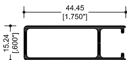
67821 CERCO PUERTA
