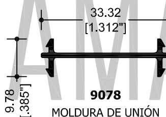
9078 MOLDURA DE UNIÓN MULLION PRODUCCIÓN SIN ACABADO
