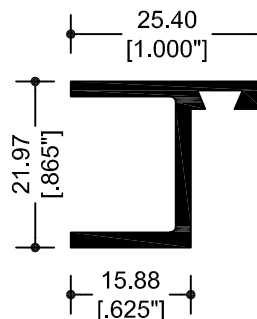
7102 BATIENTE
