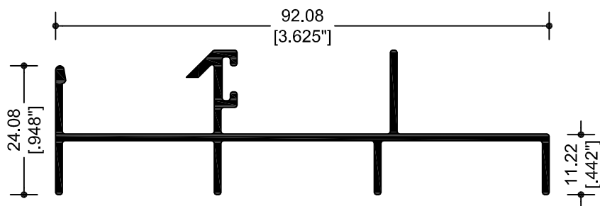
27111 JAMBA PARA CORREDIZA
