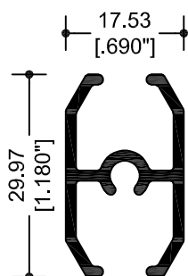
63728 PARA CUADRÍCULA RECERCADO 2"
