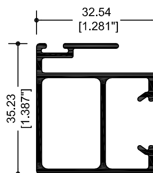
67844 CERCO TRASLAPE VENTANA
