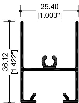
67836 CABEZAL
