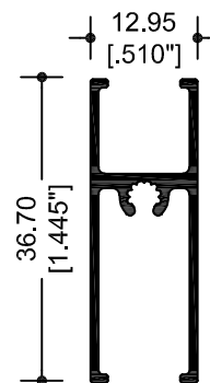
11044 CABEZAL Y ZOCLO
