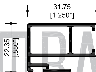
39954 TRASLAPE VENTANA
