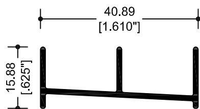
10198 RIEL INFERIOR
