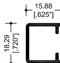
27525 CERCO FIJO ECONÓMICO
