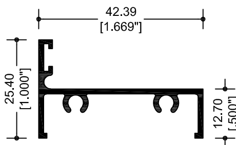
68550 MARCO PARA PUERTA
