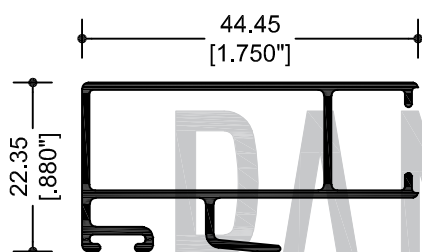
69955 TRASLAPE PUERTA
