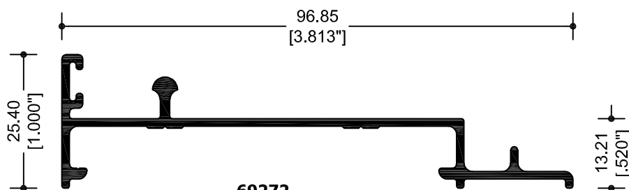
69272 RIEL PARA MOS. EXT. CORREDIZO
