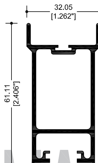
67850 CERCO OXO
