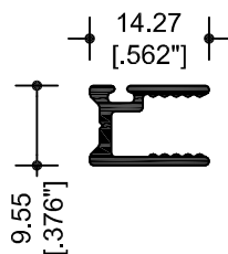
10574 CERCO FIJO
