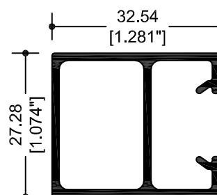
67843 CERCO VENTANA
