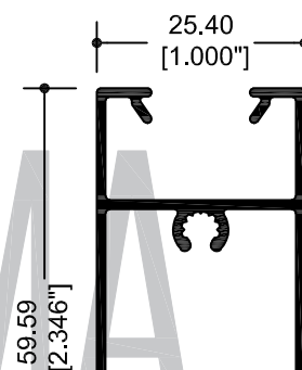
67836 CABEZAL VENTANA
