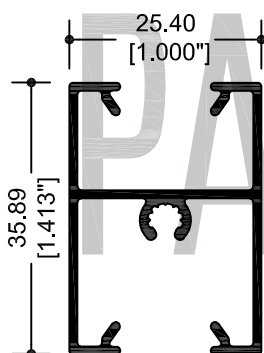
69082 INTERMEDIO
