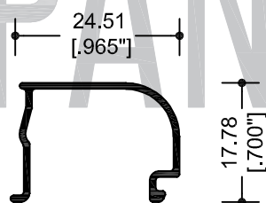
69891 JUNQUILLO CONCAVO SENCILLO (6mm)
