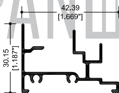
20569 RIEL
