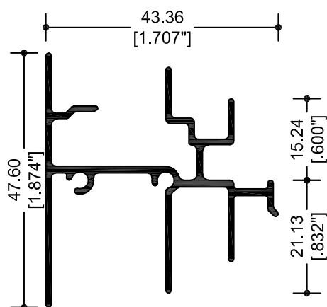
12797 RIEL Y CABEZAL
