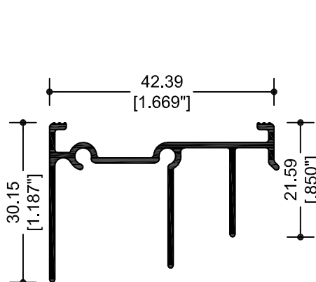
10568 CABEZAL
