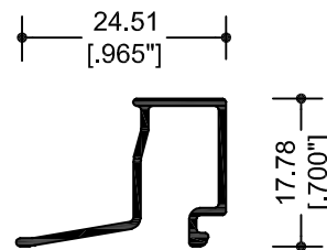
69888 JUNQUILLO CUADRADO DOBLE (18mm)
