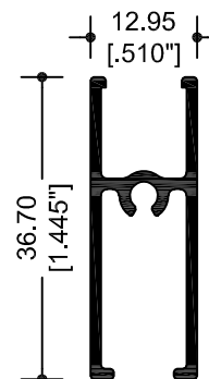
9956 CABEZAL Y ZOCLO
