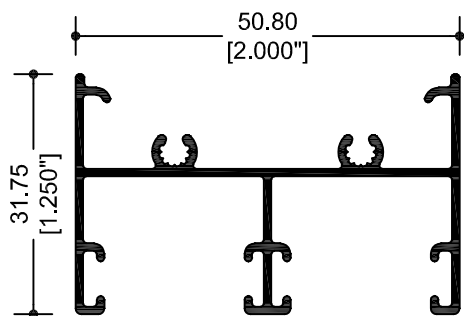
67518 CABEZAL Y JAMBA
