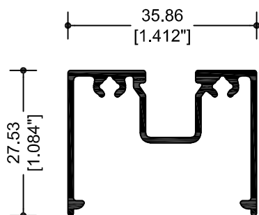
39073 BOLSA
