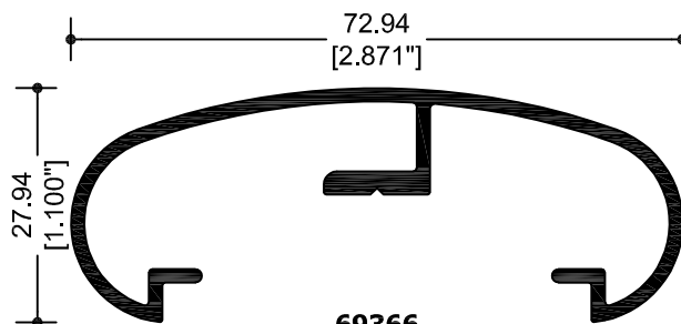
69366 PASAMANOS 3"
