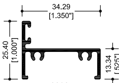
33087 MARCO PARA PUERTA
