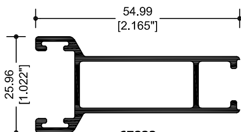
67822 CERCO OXO PUERTA
