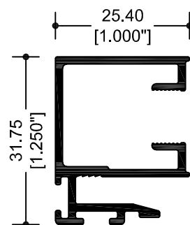
7106 CERCO TRASLAPE
