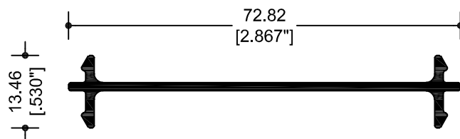
10266 MOLDURA DE UNIÓN MULLION SIN ACABADO
