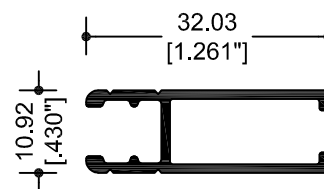
53358 ZAPATA
