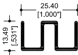
63329 GUÍA
