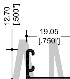
11032 BATIENTE
