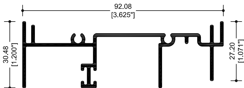
7109 CABEZAL CONTRAMARCO CORREDIZA
