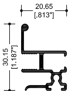
10571 CERCO MÓVIL
