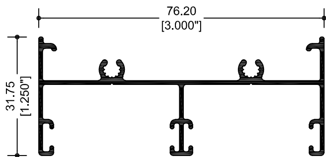
67826 CABEZAL Y JAMBA
