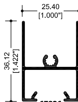
67836 CABEZAL VENTANA
