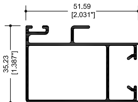
67848 TRASLAPE PUERTA
