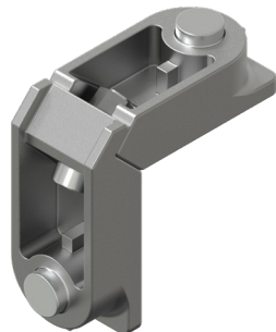
GN-650 Escuadra de botón (hoja)
