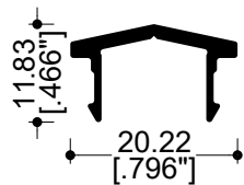
70944 Pista 2 aguas
