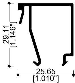
69920 Junquillo 24 mm
