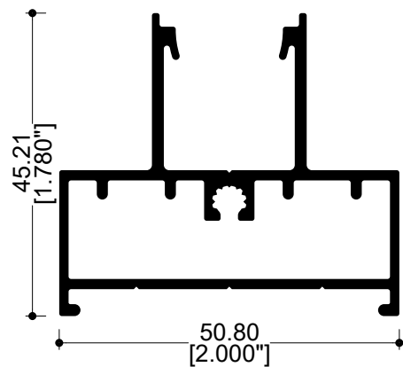
71207 Riel múltiple 45°
