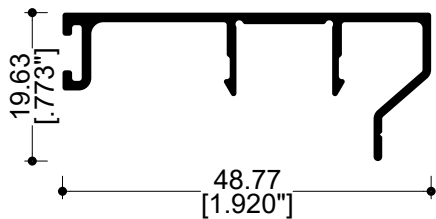
70954 Tapa vista
