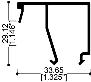
71256 Junquillo 14 mm
