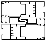
S-100 AR CLÁSICA 70947 y 70951 lxx 37.24 cm^4
