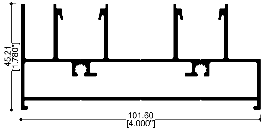
70997 Riel 2 pistas 45°
