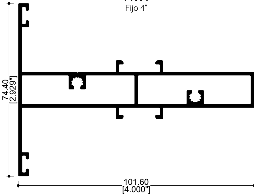
71251 Intermedio fijo
