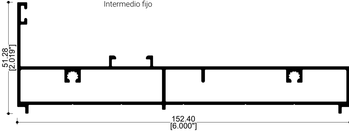
71253 Fijo 6"
