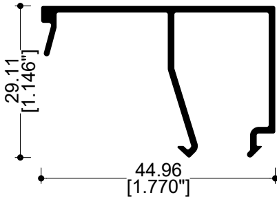
71255 Junquillo 6 mm
