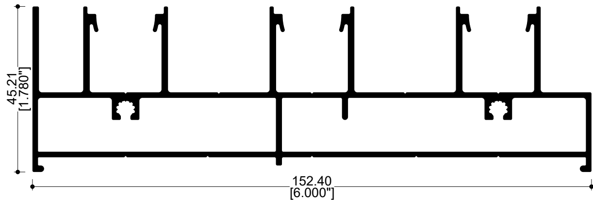
70998 Riel 3 pistas 45°
