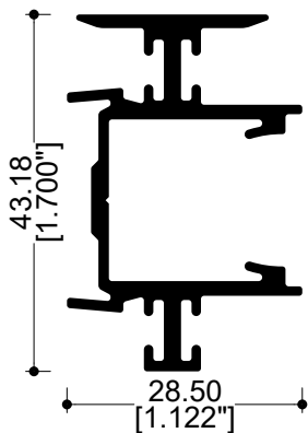
70956 Adaptador OXXO
