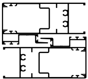
S-100 AR CLÁSICA 71205 y 70951 lxx 36.60 cm^4
