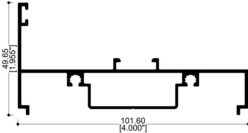
71354 Fijo 4"
