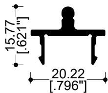
72609 Pista de gota
