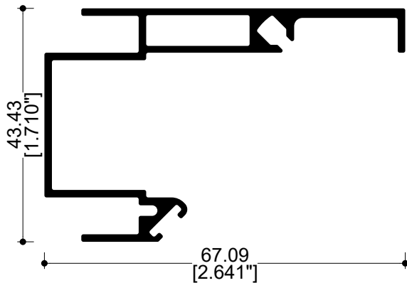
72536 Esquinero 90°
