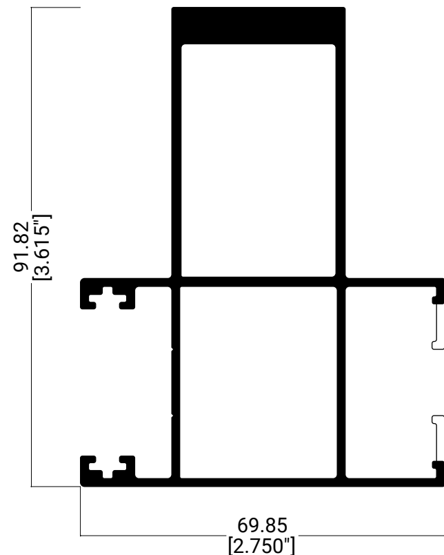
70957 Cerco reforzado 6 mm
