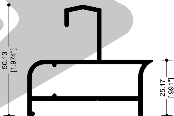
62091 ADAPTADOR RIEL
