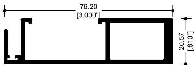
72535 TRASLAPE PANORÁMICO 3"
