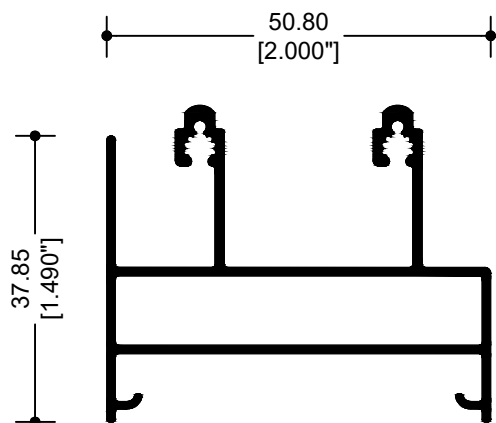
68842 RIEL
