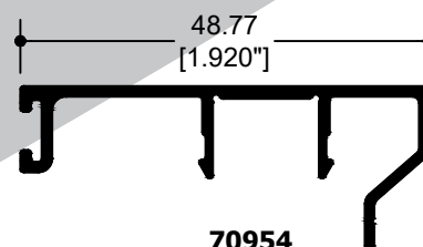
70954 TAPA VISTA
