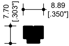
14412 CONECTOR P/REFUERZO
