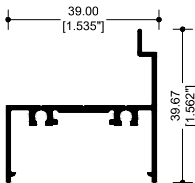
13363 CONTRAMARCO
