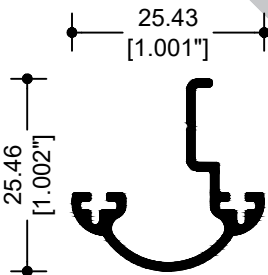
12653 ADAPTADOR INTERMEDIO
