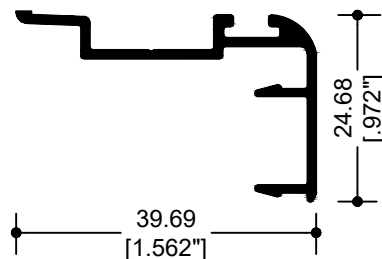
67899 TRASLAPE PUERTA
