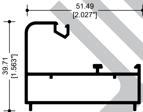
62079 ESCALONADO
