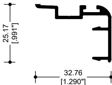
62070 TRASLAPE VENTANA
