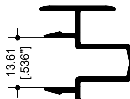
62103 OXXO
