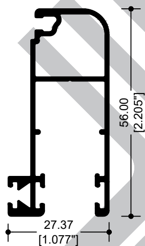
68337 MOSQUITERO BAJO
