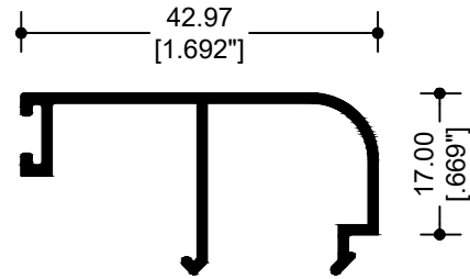
62022 JUNQUILLO
