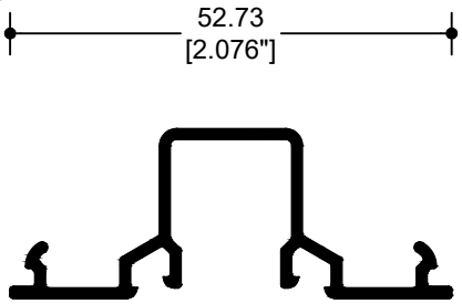
12505 TAPA BOLSA
