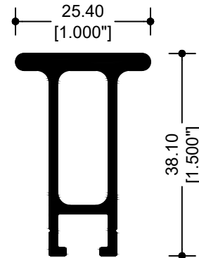
14411 REFUERZO 1 1/2"
