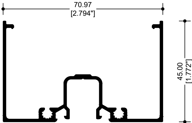
22504 BOLSA
