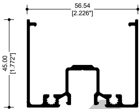
12504 BOLSA
