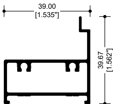
12273 CONTRAMARCO
