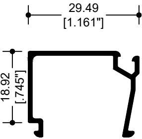
42507 JUNQUILLO
