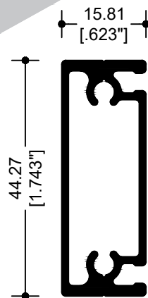
11411 MOSQUITERO
