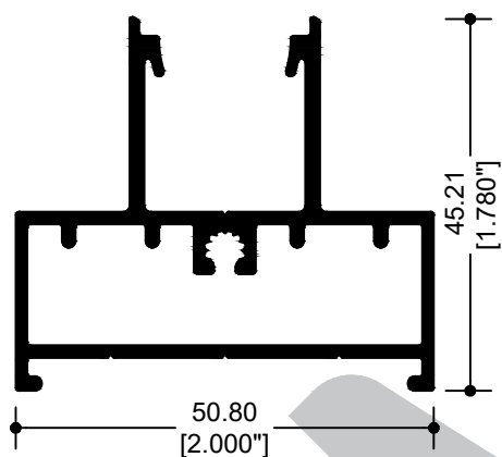
71207 RIEL MÚLTIPLE 45°
