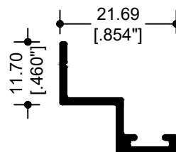
50701 ADAPTADOR OXXO
