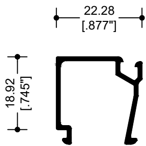
12507 JUNQUILLO
