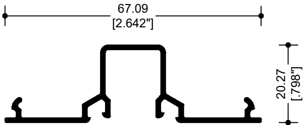
42505 TAPA BOLSA
