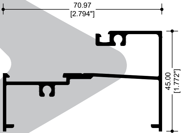
22513 ESCALONADO INTERIOR
