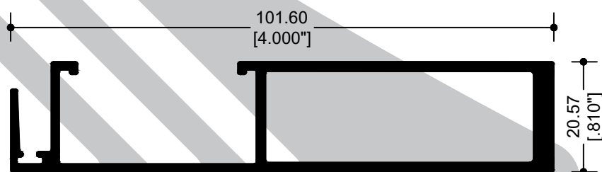
72610 TRASLAPE PANORÁMICO 4"
