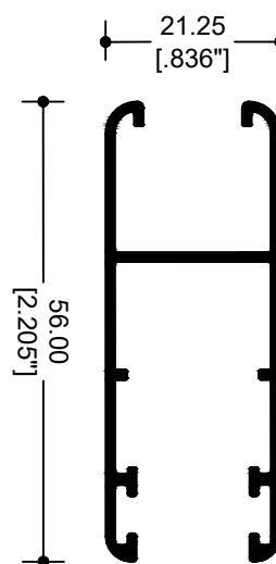
62066 CERCO
