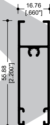
68843 ZOCLO
