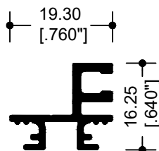
69368 ADAPTADOR MOSQUITERO
