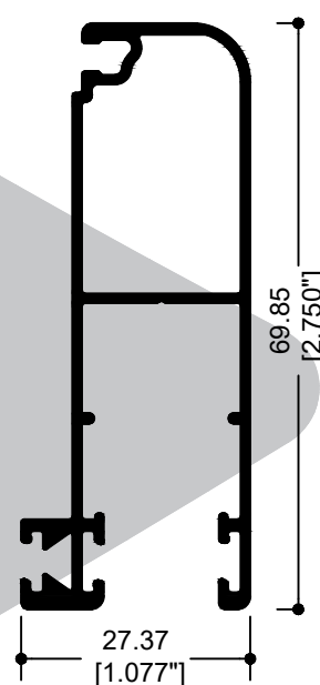
68299 MOSQUITERO EXT.
