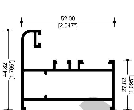
62033 "L" CONTRAMARCO
