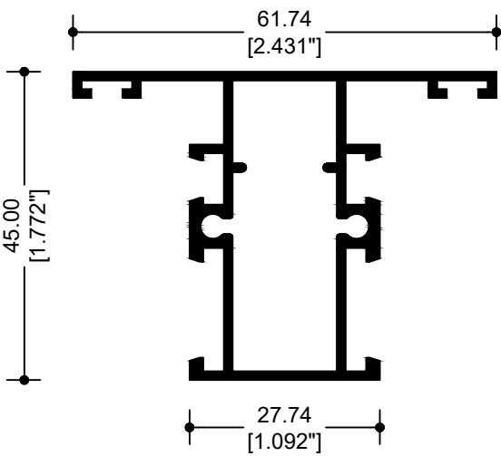
62041 INTERMEDIO CUADRÍCULA
