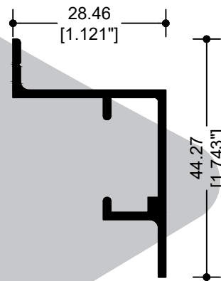
11409 CABEZAL MOSQUITERO
