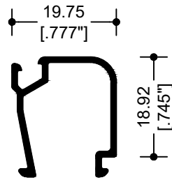
62072 JUNQUILLO
