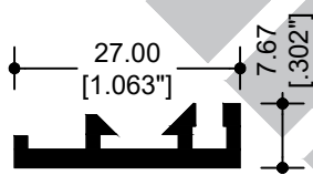
5173 MOSQUITERO
