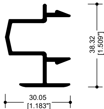
64206 ADAPTADOR OXXO
