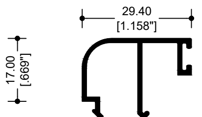
62029 JUNQUILLO 6mm.
