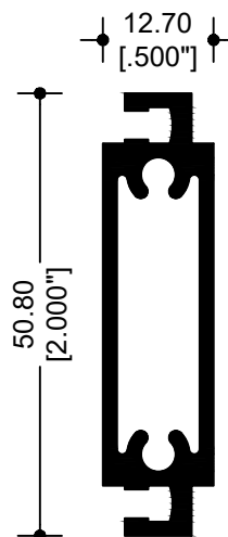
7101 MOSQUITERO INTERMEDIO
