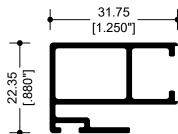
39954 TRASLAPE VENTANA
