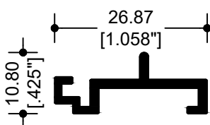
9966 ADAPTADOR MOSQUITERO
