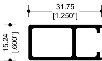
8320 CERCO VENTANA
