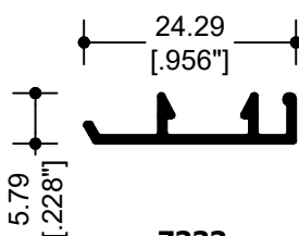
7333 MOSQUITERO
