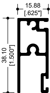
10358 MOSQUITERO
