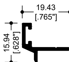
10220 ADAPTADOR OXXO
