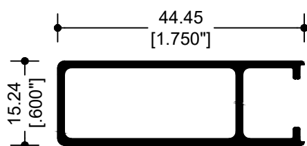
67821 CERCO PUERTA
