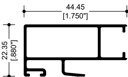
69955 TRASLAPE PUERTA
