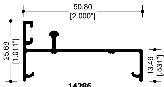
14286 RIEL
