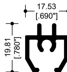
63727 BARROTILO 2"
