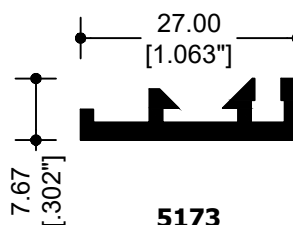
5173 MOSQUITERO
