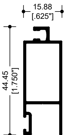
66534 CERCO MOSQUITERO
