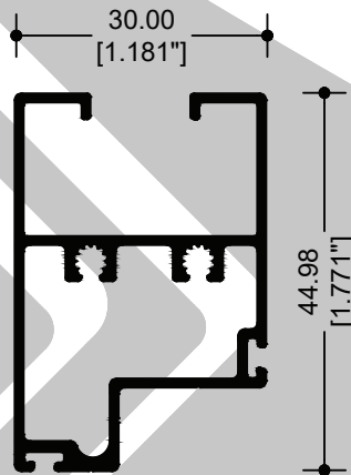
12276 MARCO
