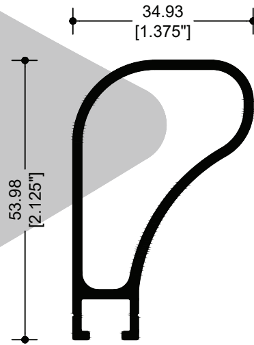
62014 REFUERZO
