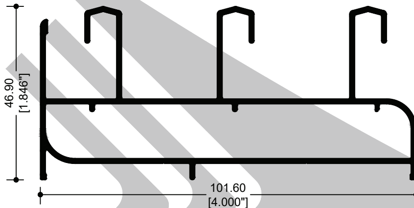
82017 MARCO 3 VÍAS
