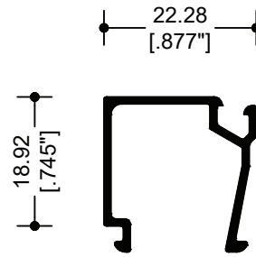
12507 JUNQUILLO
