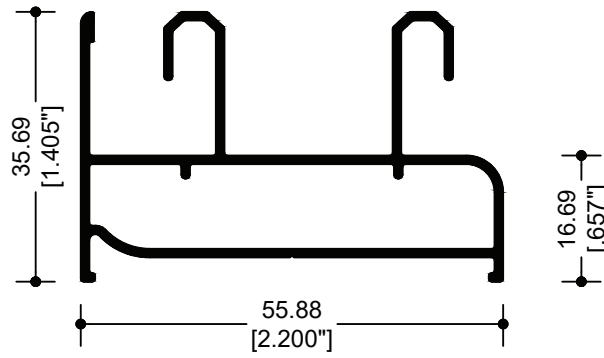
87896 MARCO 2 VIAS S-60
