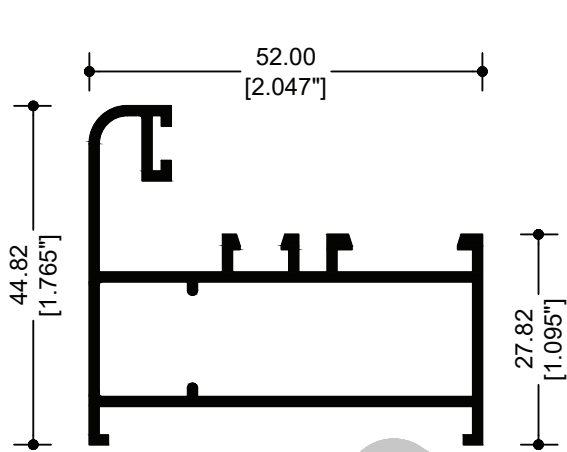
62033 "L" CONTRAMARCO
