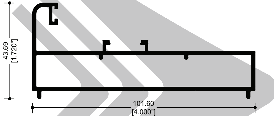
87734 FIJO 4"
