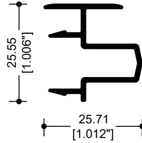
82103 ADAPTADOR OXXO
