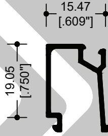
12543 JUNQUILLO
