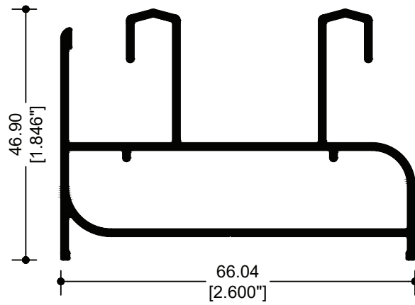
82000 MARCO 2 VÍAS
