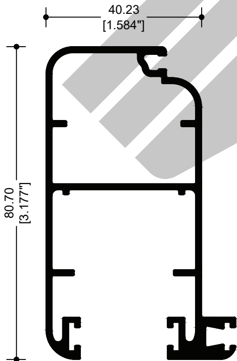
62057 MOSQUITERO
