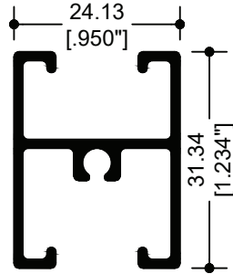
12456 INTERMEDIO
