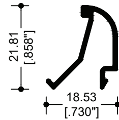
82030 JUNQUILLO VIDRIO DOBLE
