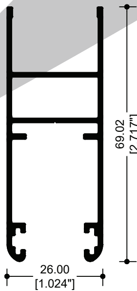
82004 HOJA DE VIDRIO DOBLE
