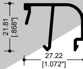
82029 JUNQUILLO VIDRIO SENCILLO
