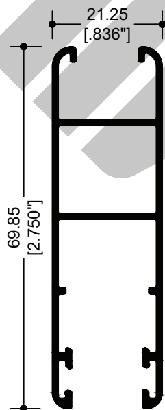
67894 CERCO PUERTA
