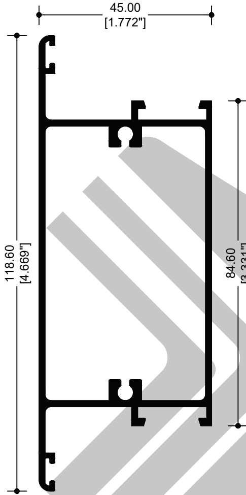
62039 INTERMEDIO
