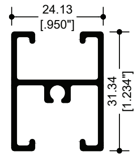
12456 INTERMEDIO
