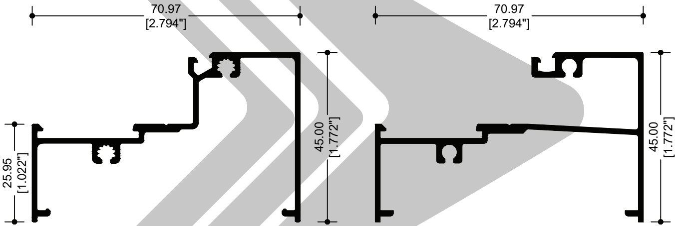
32506 ESCALONADO EXTERIOR
