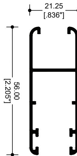
62066 CERCO VENTANA
