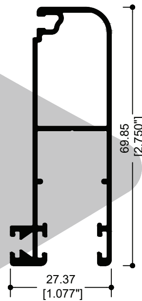
68299 MOSQUITERO EXT.
