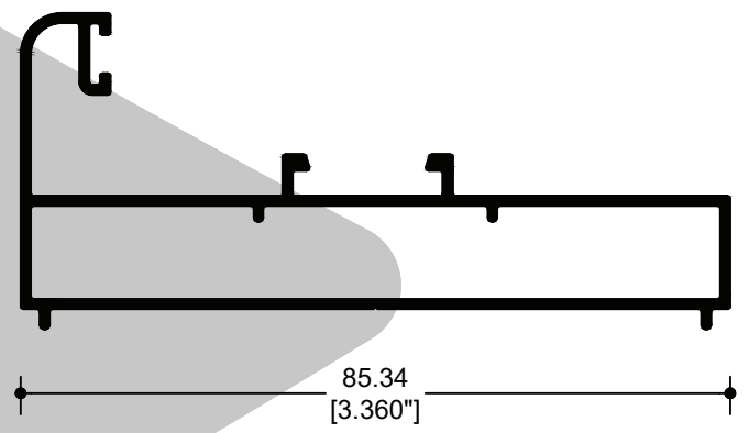
82093 FIJO 3 VIAS S-60
