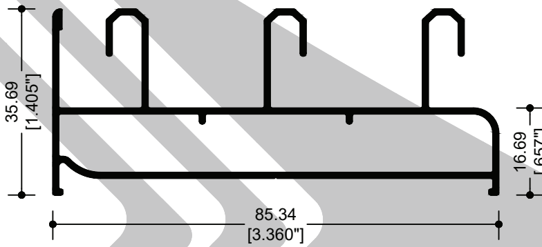
88300 MARCO 3 VIAS S-60
