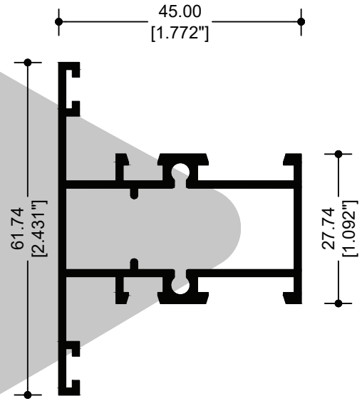
62041 INTERMEDIO CUADRÍCULA
