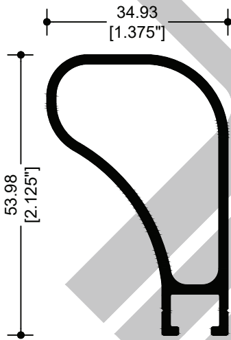
62014 REFUERZO
