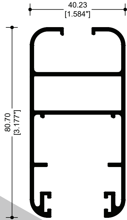
62055 CERCO 6mm
