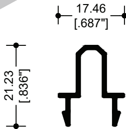
62078 ADAPTADOR XX
