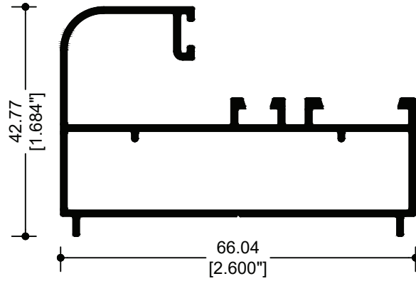
82092 FIJO
