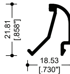
82030 JUNQUILLO VIDRIO DOBLE
