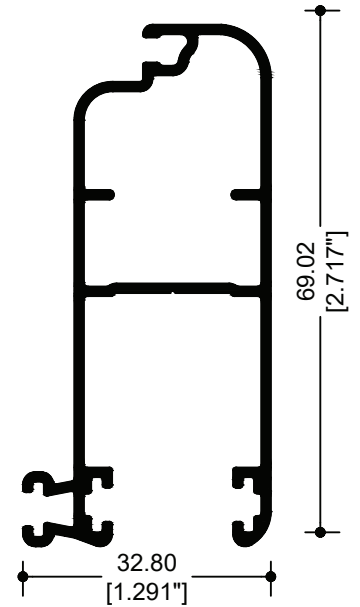
82019 MOSQUITERO
