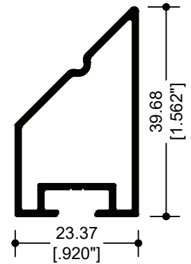
71643 MC ESQUINERO 90-270
