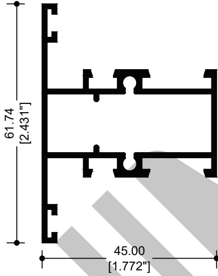
62041 INTERMEDIO CUADRÍCULA
