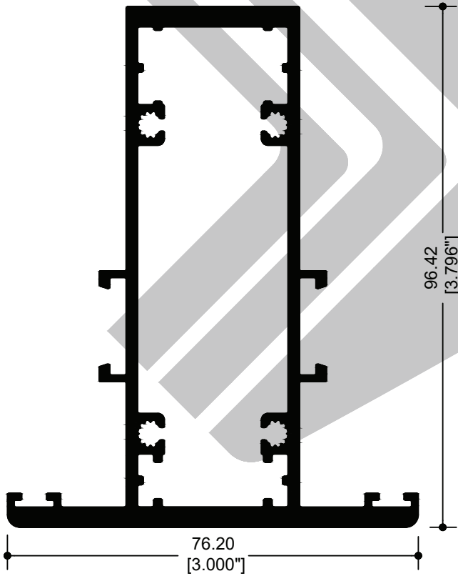
87735 INTERMEDIO
