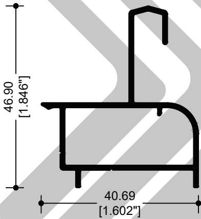
84207 PISTA ADICIONAL
