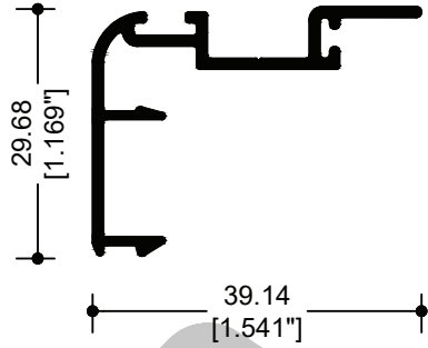
82002 TRASLAPE
