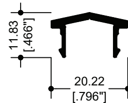
70944 PISTA 2 AGUAS
