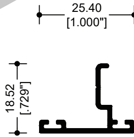
74272 ADAPTADOR INTERMEDIO PLANO
