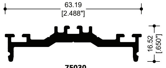
75030 MCM MOLDURA UNIÓN SDN 10MM Y 31MM
