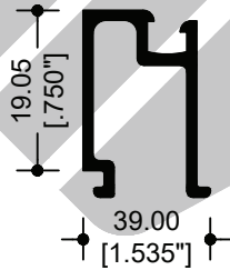
12609 JUNQUILLO
