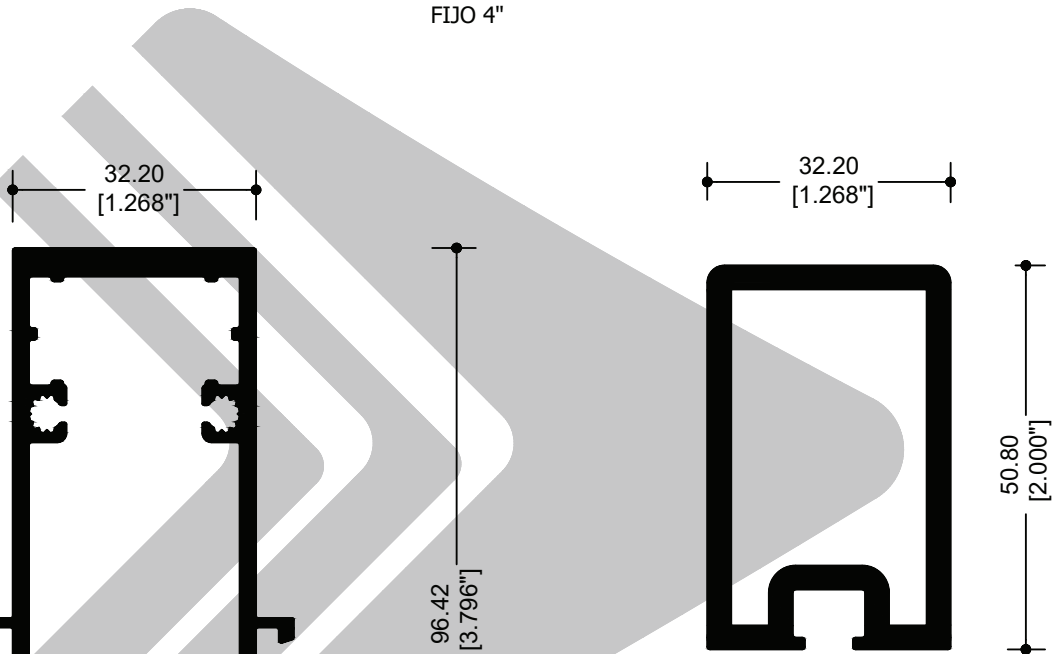
67712 REFUERZO PARA INTERMEDIO
