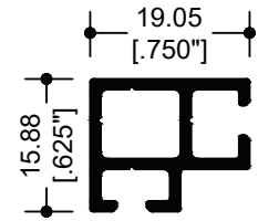
71527 MCM ADAPTADOR 9 ó 6
