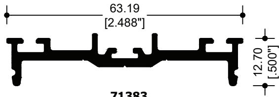
71383 MCM MOLDURA UNIÓN 6MM Y 24MM
