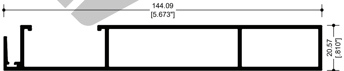
71254 TRASLAPE ESBELTO
