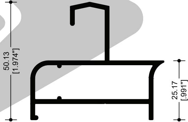
62091 ADAPTADOR RIEL
