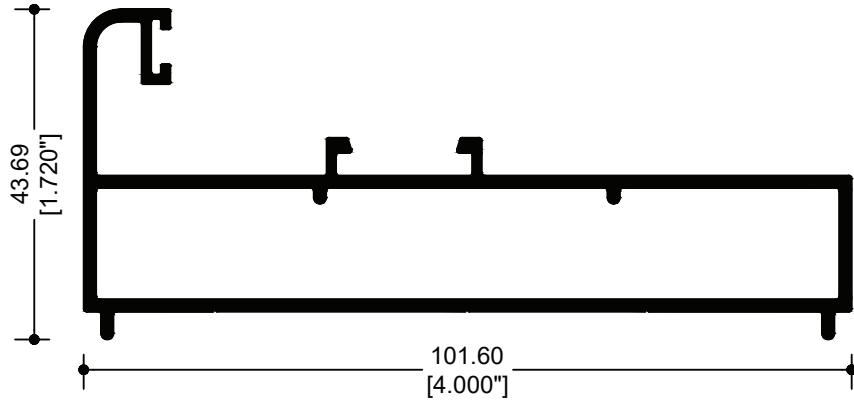
87734 FIJO 4"
