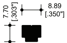
14412 CONECTOR P/REFUERZO
