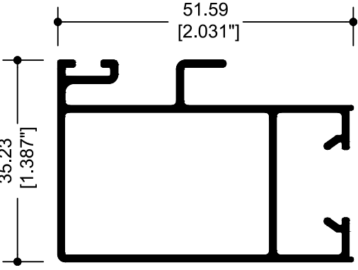
67848 TRASLAPE PUERTA
