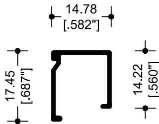
36370 JUNQUILLO
