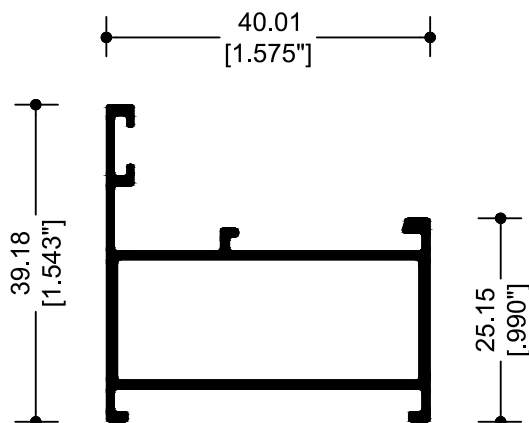
69877 MARCO VENTANA
