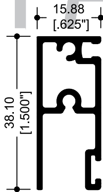
10358 MOSQUITERO
