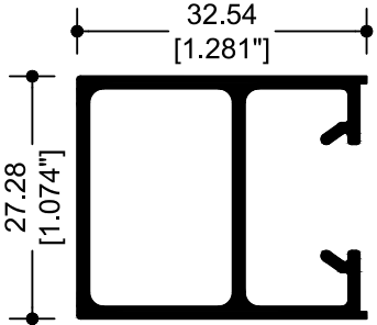
67843 CERCO VENTANA
