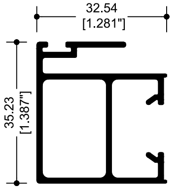
67844 CERCO TRASLAPE VENTANA
