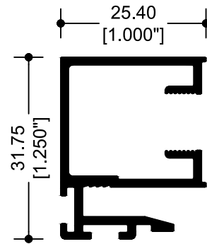
7106 CERCO TRASLAPE
