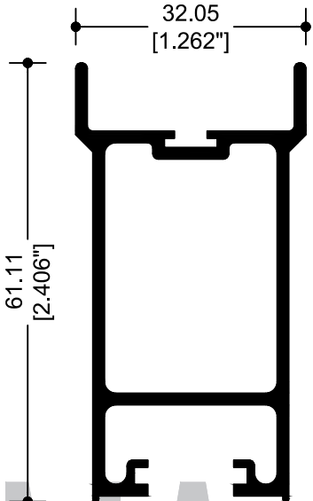
67850 CERCO OXXO
