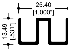
63329 GUÍA
