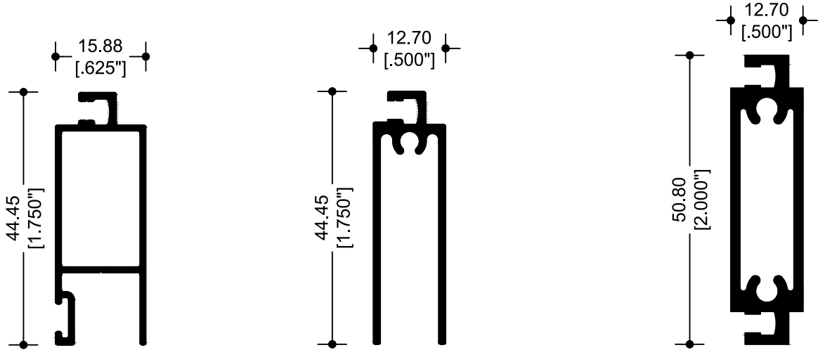
66534 CERCO MOSQUITERO
