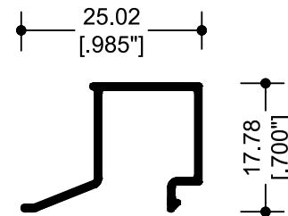
74635 JUNQUILLO ESTRECHO
