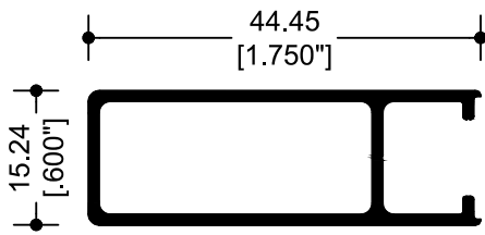
67821 CERCO PUERTA
