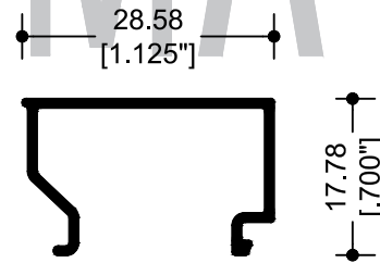
73978 JUNQUILLO ANCHO
