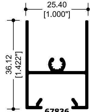
67836 CABEZAL VENTANA
