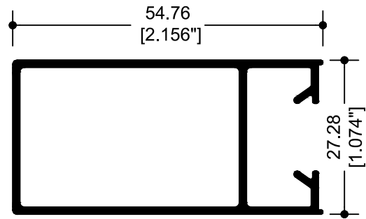
9236 CERCO CHAPA
