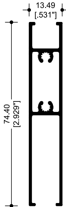
37825 ZOCLO PUERTA
