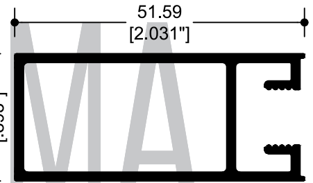
7105 CERCO CHAPA
