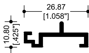
9966 ADAPTADOR MOSQUITERO
