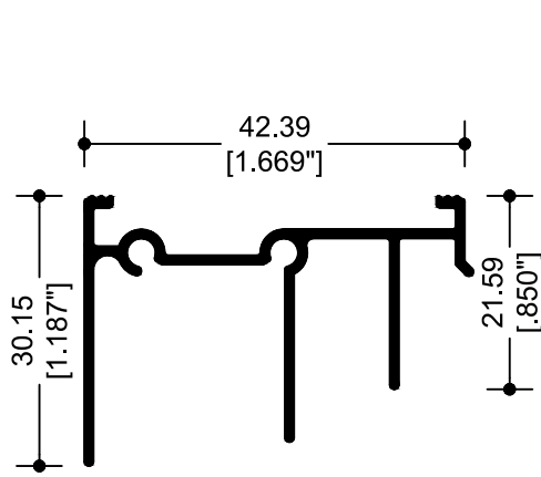
10568 CABEZAL
