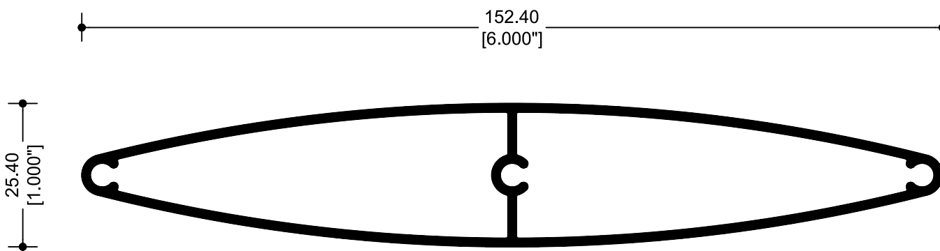
67362 CELOSÍA 6" PRODUCCIÓN
