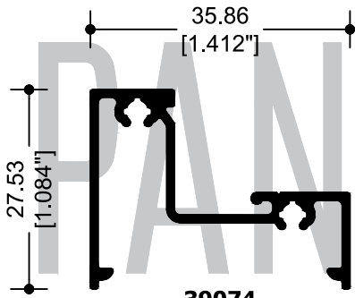
39074 ESCALONADO
