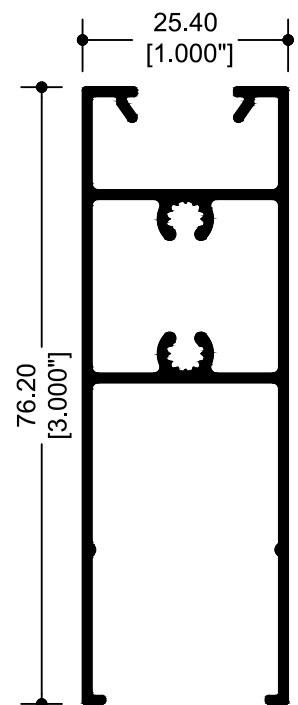
67842 ZOCLO
