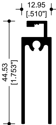
7104 MOSQUITERO
