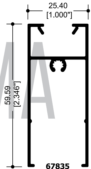
67835 ZOCLO VENTANA
