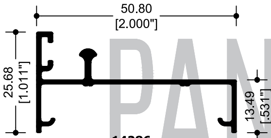
14286 RIEL
