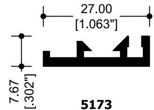
5173 MOSQUITERO
