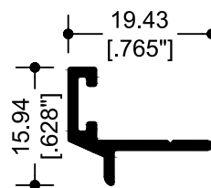
10220 ADAPTADOR OXXO
