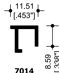
7014 JUNQUILLO
