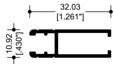
53358 ZAPATA
