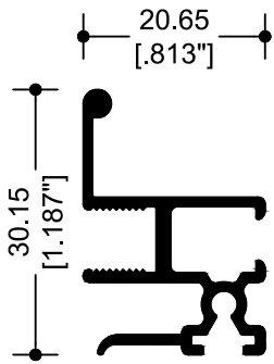
10571 CERCO MÓVIL
