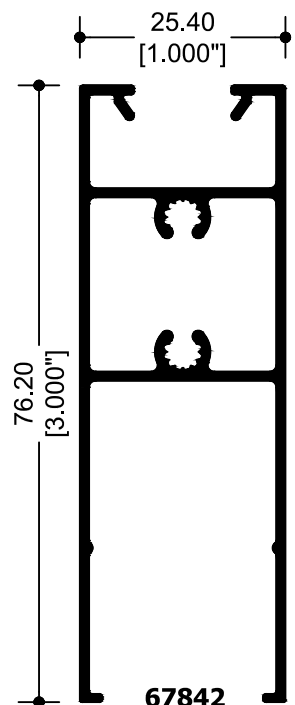
67842 ZOCLO PUERTA
