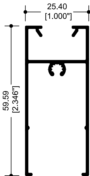
67835 ZOCLO
